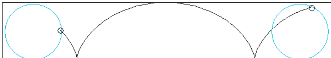
Figure 8-131 サイクロイド( Cycloid :幾何学模様的一种)
