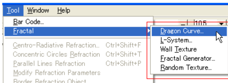
Figure 10-57 フラクタル図形(Fractal graphics)
